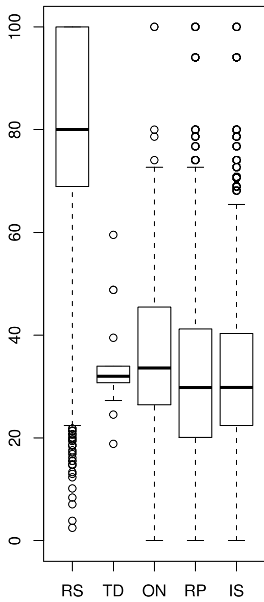
(D) Partial Donor (+3 to +6)
